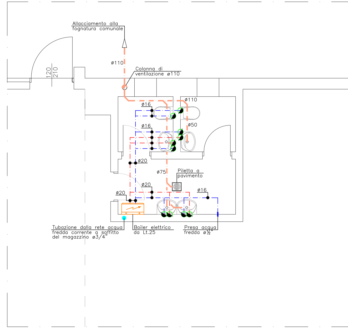
– BLOCCO BAGNI "5B" – IMPIANTO IDRICO-SANITARIO
