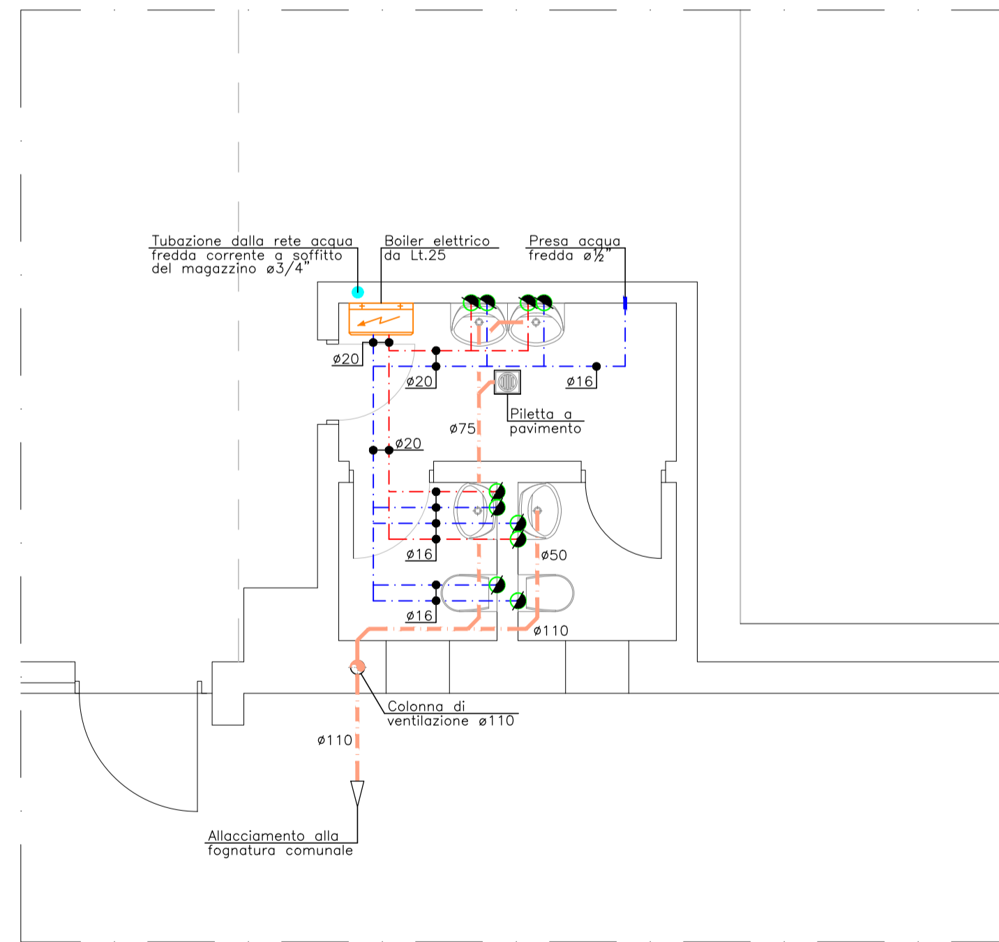
– BLOCCO BAGNI "2B" – IMPIANTO IDRICO-SANITARIO
