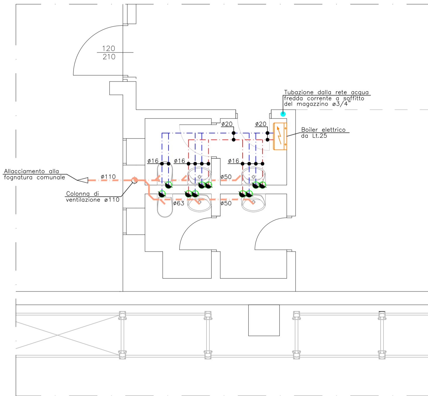
– BLOCCO BAGNI "1B" – IMPIANTO IDRICO-SANITARIO
