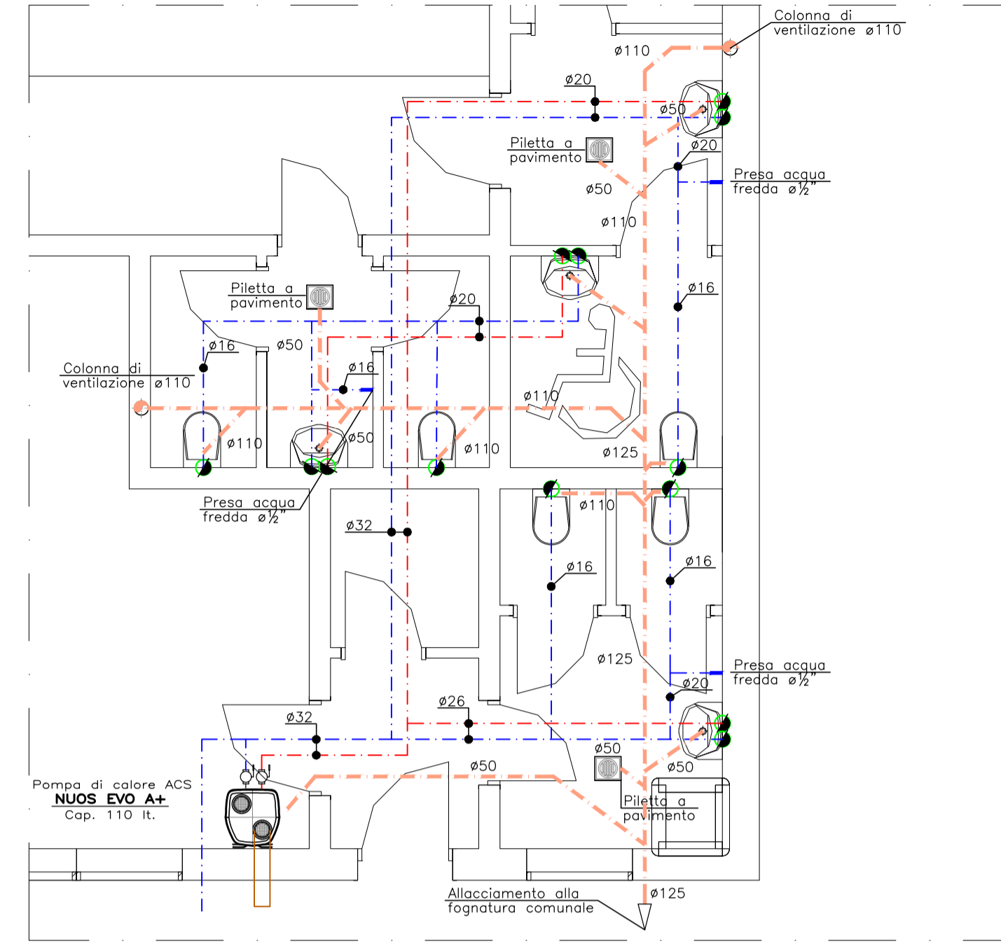
– BLOCCO BAGNI "6C" – IMPIANTO IDRICO-SANITARIO
