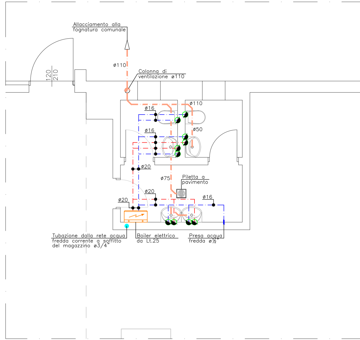
– BLOCCO BAGNI "4B" – IMPIANTO IDRICO-SANITARIO
