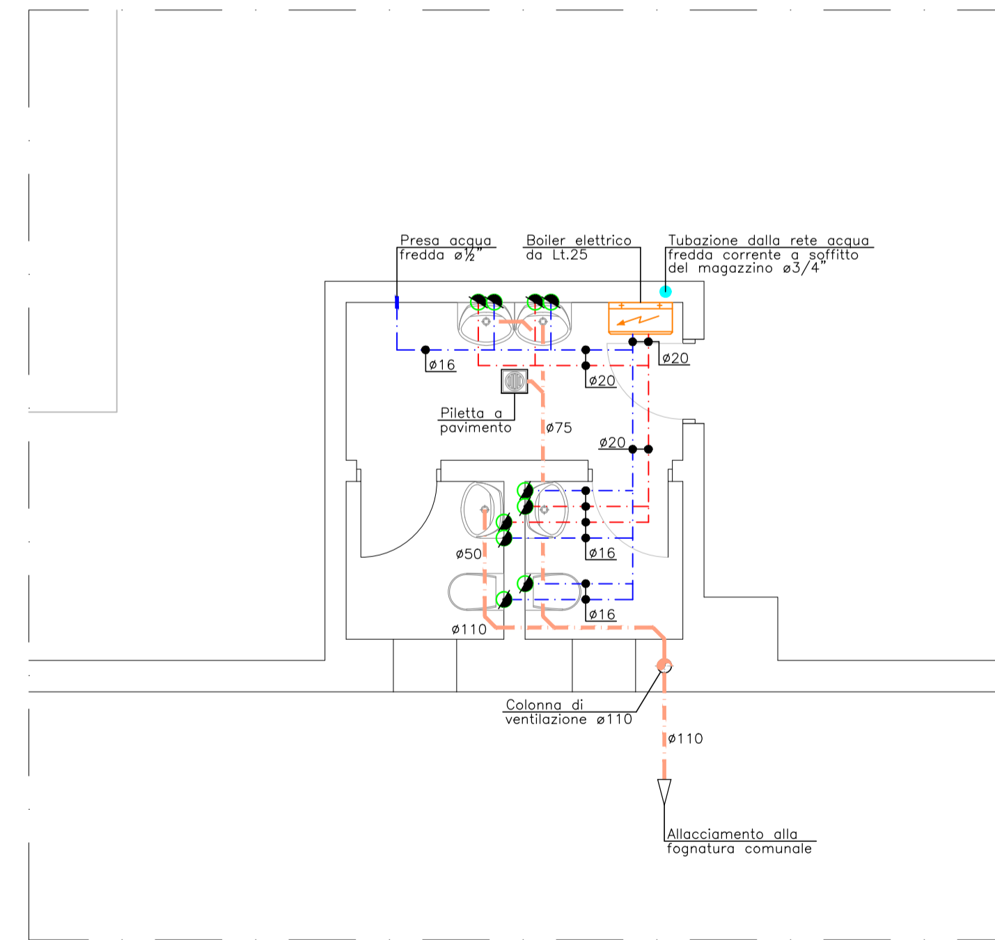
– BLOCCO BAGNI "3B" – IMPIANTO IDRICO-SANITARIO
