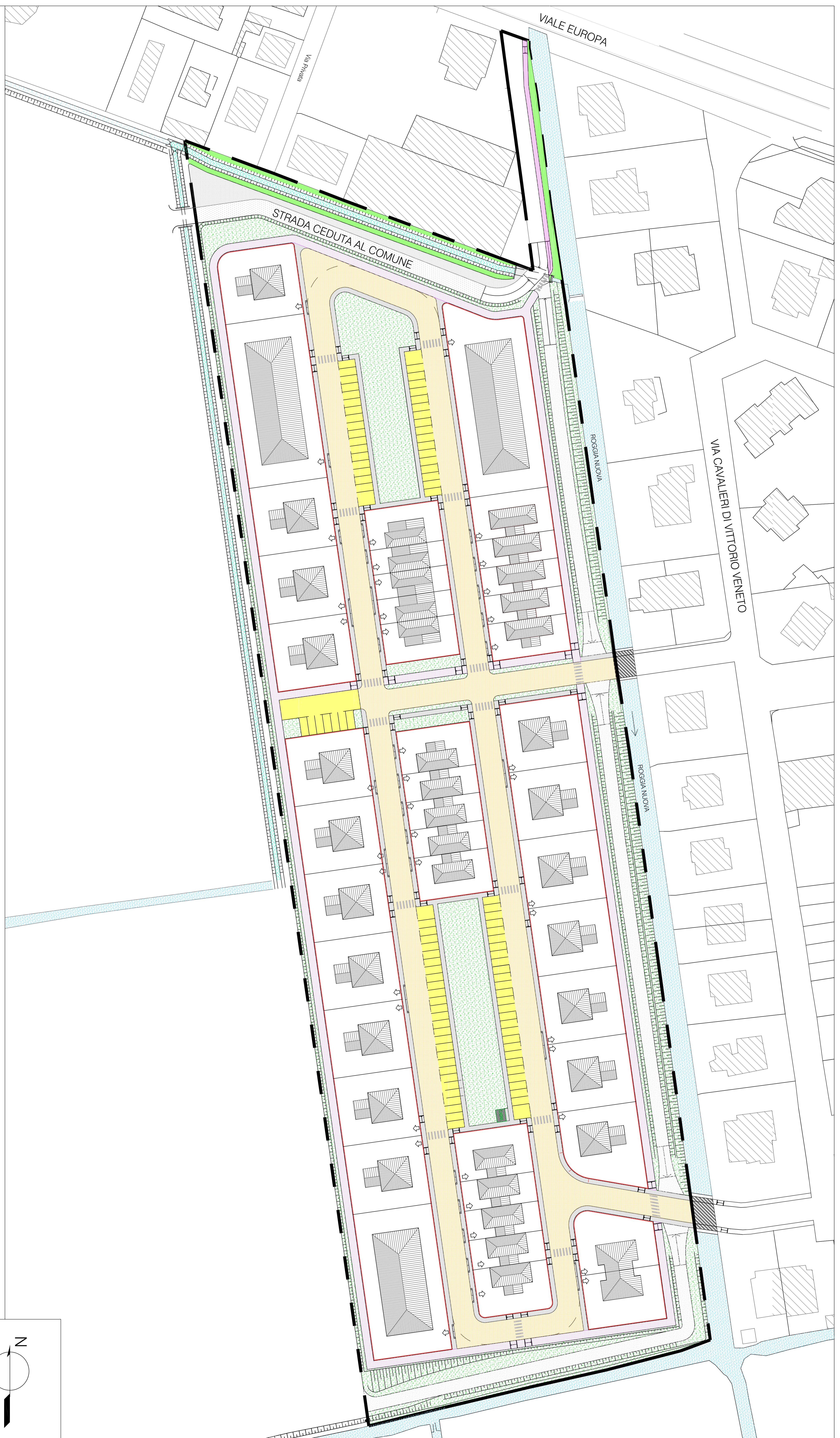
PLANIMETRIA SCALA 1:500
